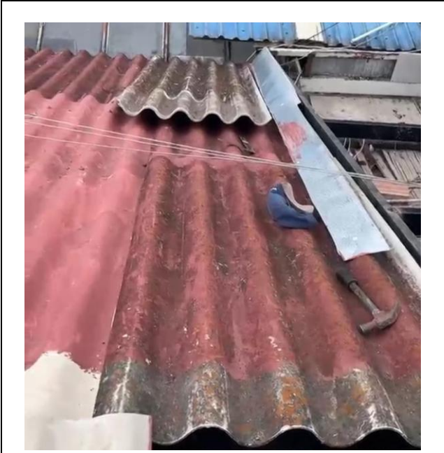
DESMONTE TEJA
